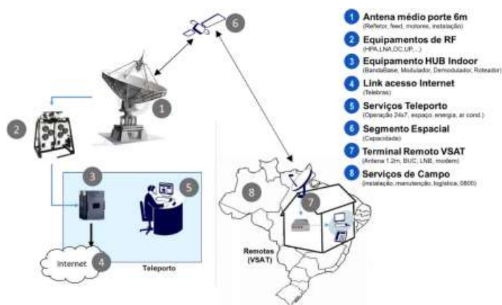
Figura 8 - Componentes do sistema de comunicação via satélite
